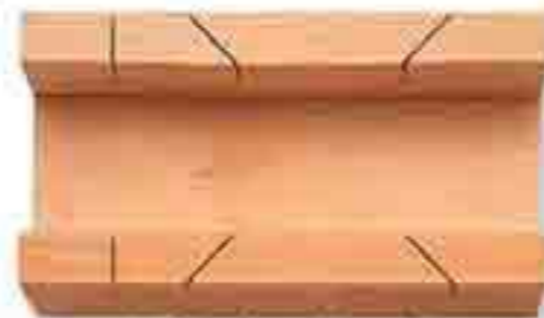
قالب القطع المائل qaalib al-qata al-maa'il miter block
